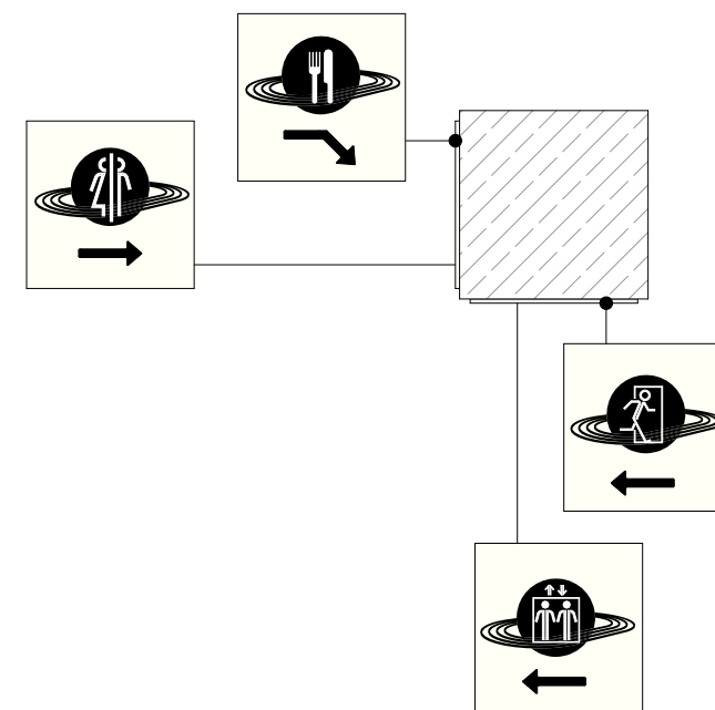
WARIANT G 4 TABLICZKI ZAWIESZONE NA SŁUPIE
